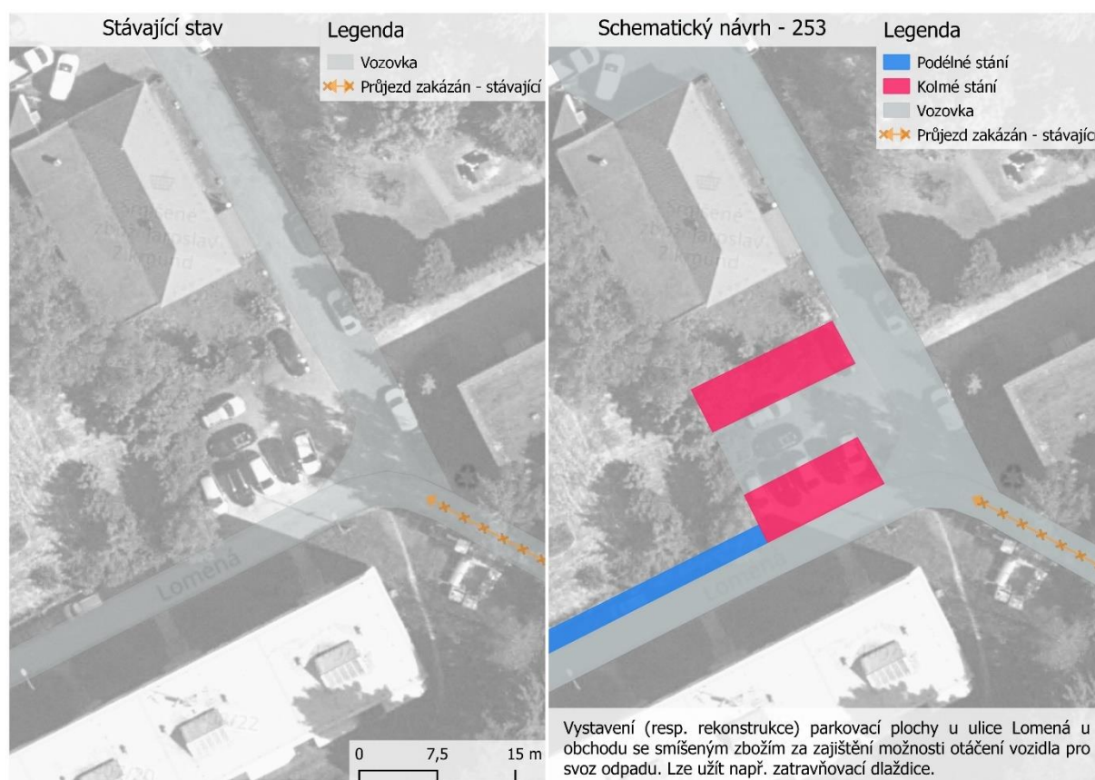
Obrázek 4.55: Schematické znázornění navrhovaného opatření č. 253.
