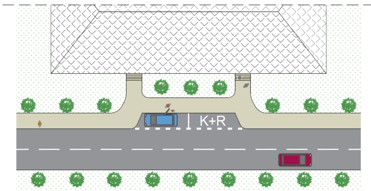
Obrázek 4.118: Záliv typu K+R – schéma.
