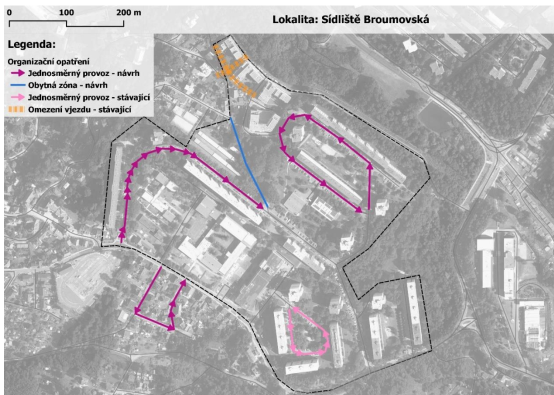
Obrázek 4.96: Schematické znázornění návrhu organizace dopravy na sídlšti Broumovská.
