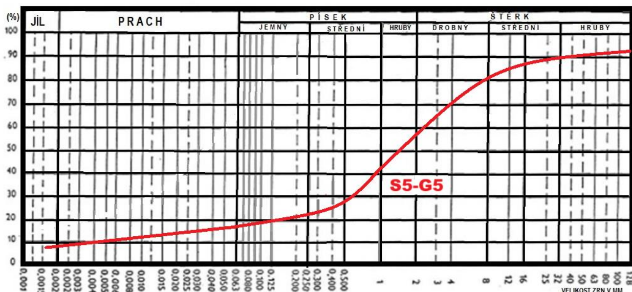
křivky zrnitosti vzorků zemin č. 125 2025
